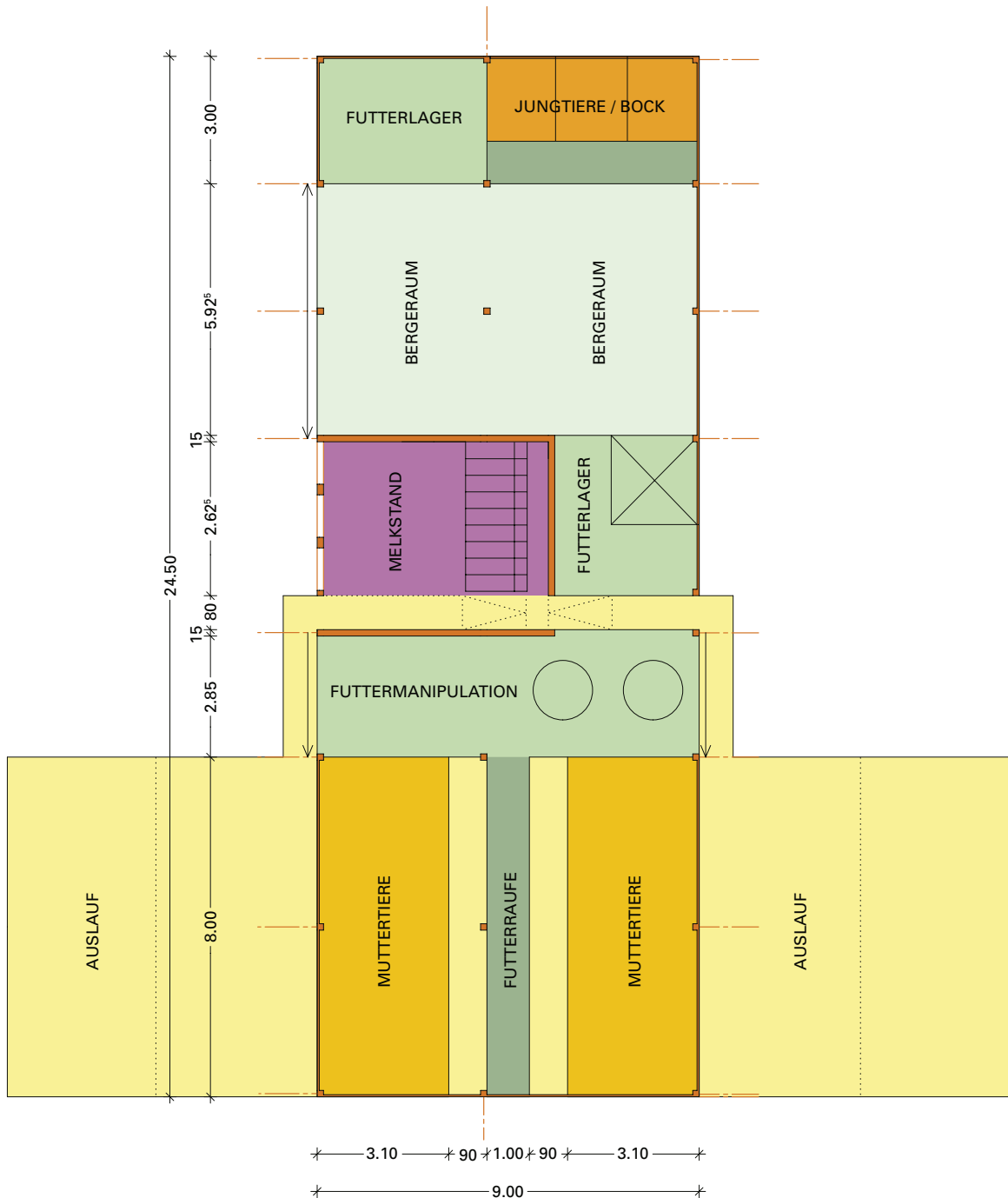
GRUNDRISS
